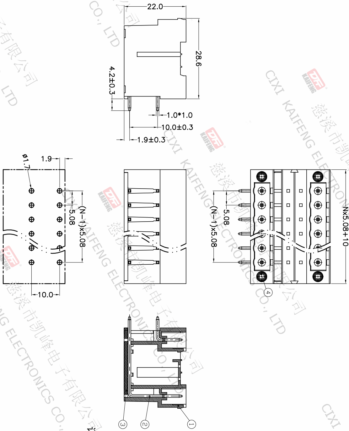
P.C.B. LAYOUT
