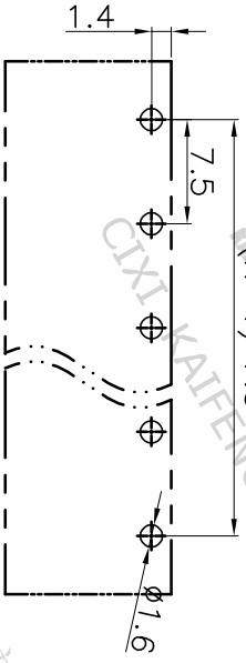
P.C.B.LAYOUT
